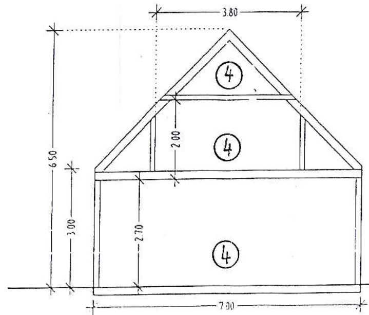
SCHNITT GARAGE
